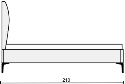
BED 160X200
