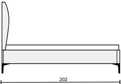
BED 135X190
